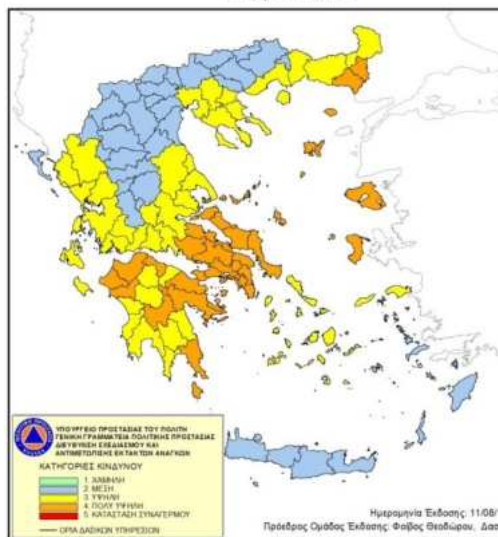
ΧΑΡΤΗΣ ΠΡΟΒΛΕΨΗΣ ΚΙΝΔΥΝΟΥ ΠΥΡΚΑΓΙΑΣ ΠΟΥ ΙΣΧΥΕΙ Δευτέρα 12/08/19
